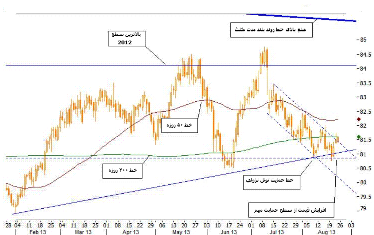
نمودار روند تغییرات روزانه شاخص جهانی ایندکس دلار آمریکا
